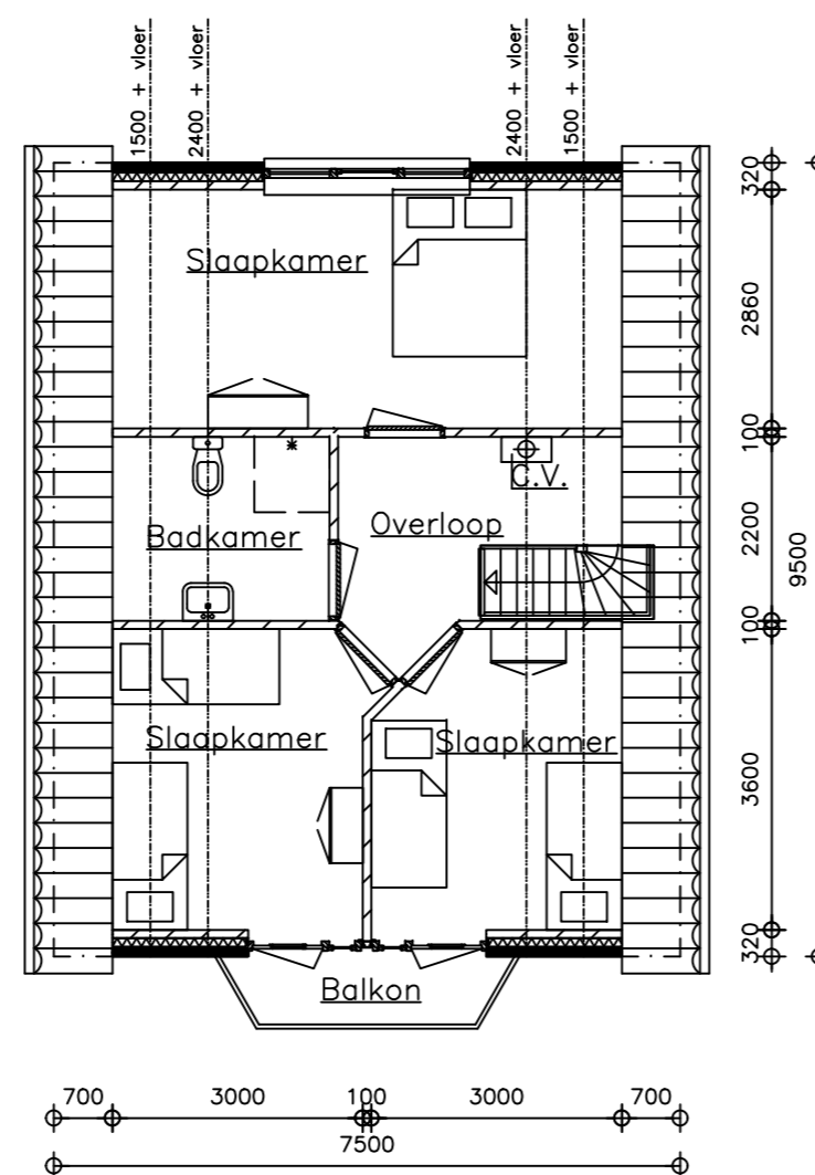
Verdieping
