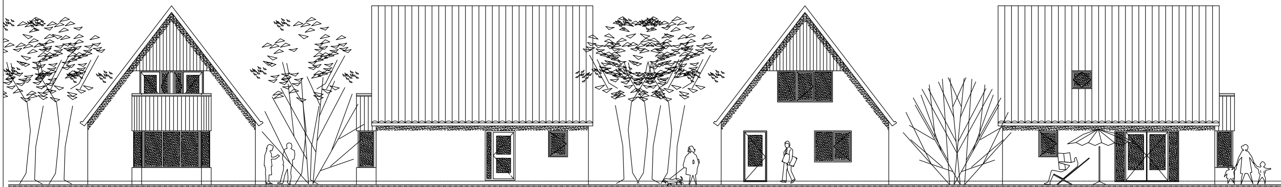
Voorgevel
