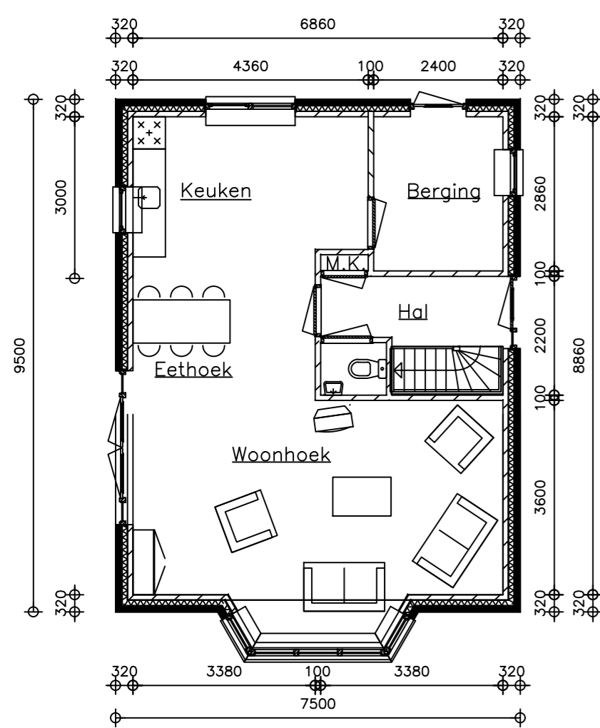
Begane grond
