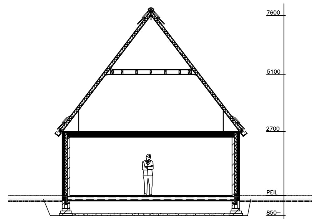
Doorsnede
